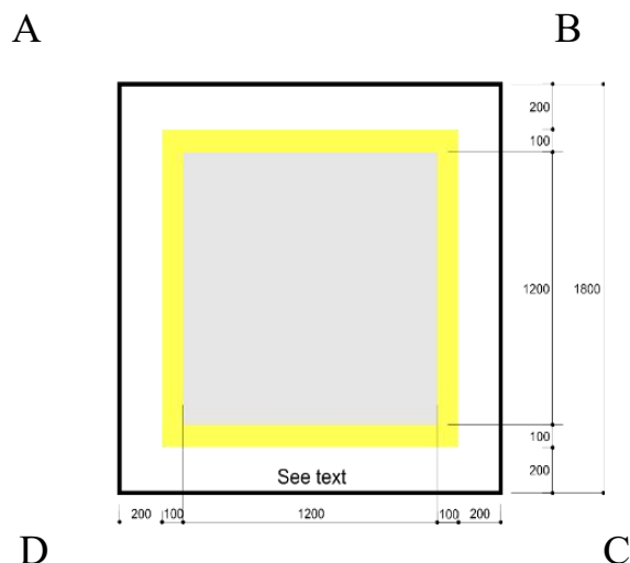
Рисунок № 1.2. Размеры ковра для вольных упражнений
