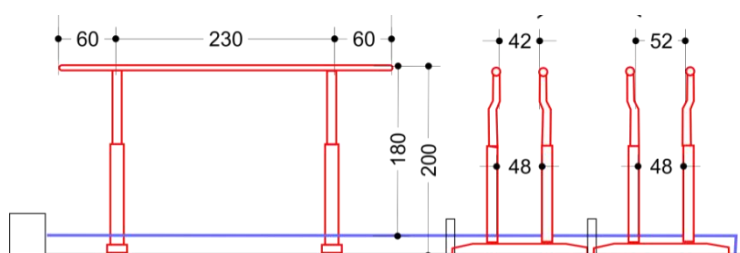
Рисунок № 1.8. Размеры параллельных брусьев
