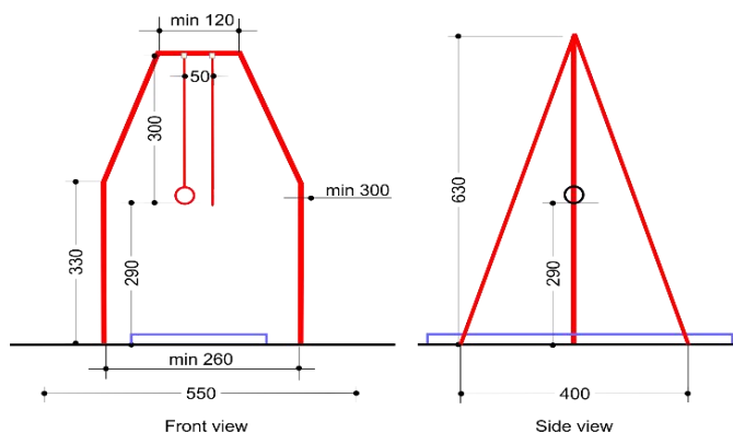
Рисунок № 1.4. Размеры колец
