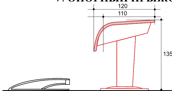
Рисунок № 1.5. Размеры стола для опорного прыжка.
