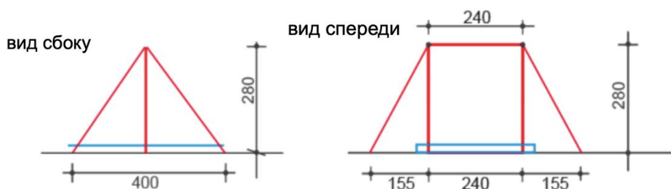
Рисунок № 1.9. Размеры перекладины
