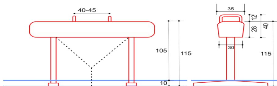
Рисунок № 1.3. Размеры коня
